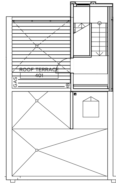
ROOFTOP SCALE: 1/8" = 1'-0" TYPE B - WEST
